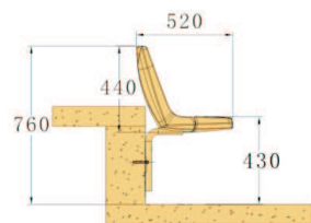
Kotvení do boku stupně
